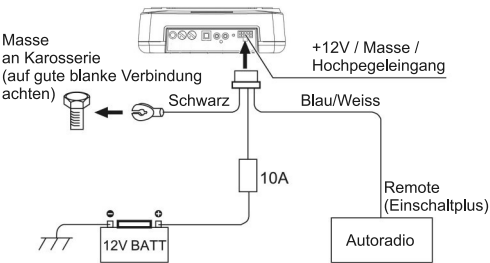
Anschlussdiagramm
