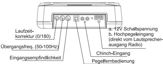
Funktionskontrolldiagramm
