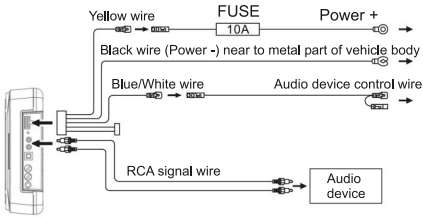
Anschlussdiagramm 2 (Chinch-Eingang)
