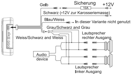
Anschlussdiagramm 1 (Hochpegel)
